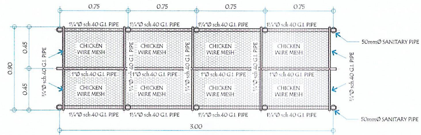
PLAN SCALE: 1 : 25m
