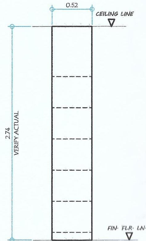
END ELEVATION (CABINET-1) SCALE: 1:30 M
