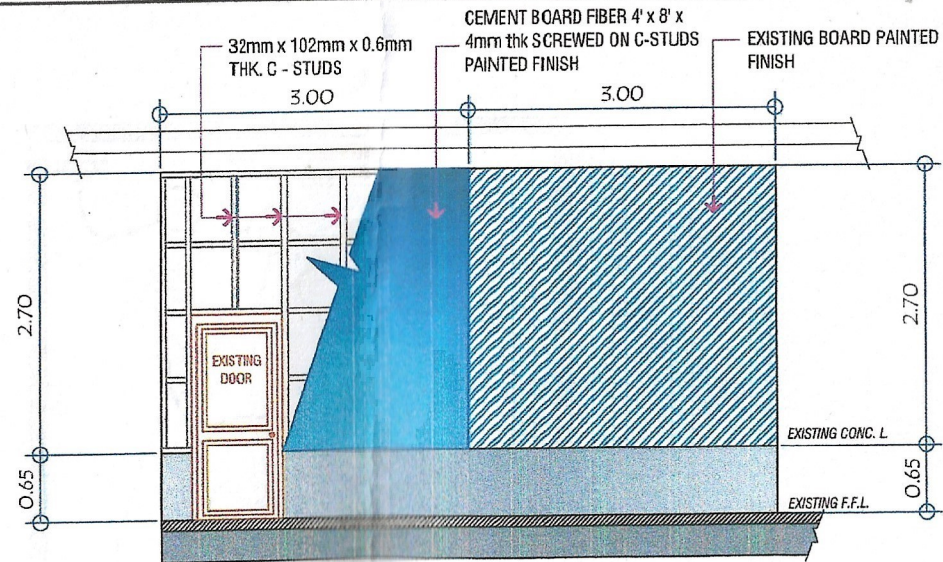
RIGHT SIDE ELEVATION SCALE: 14 : 1 M
