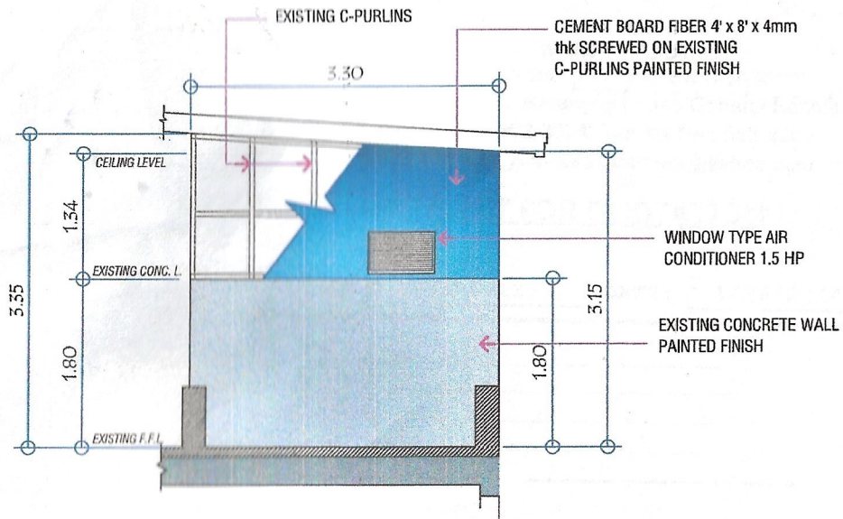
REAR ELEVATION SCALE: 14 : 1 M
