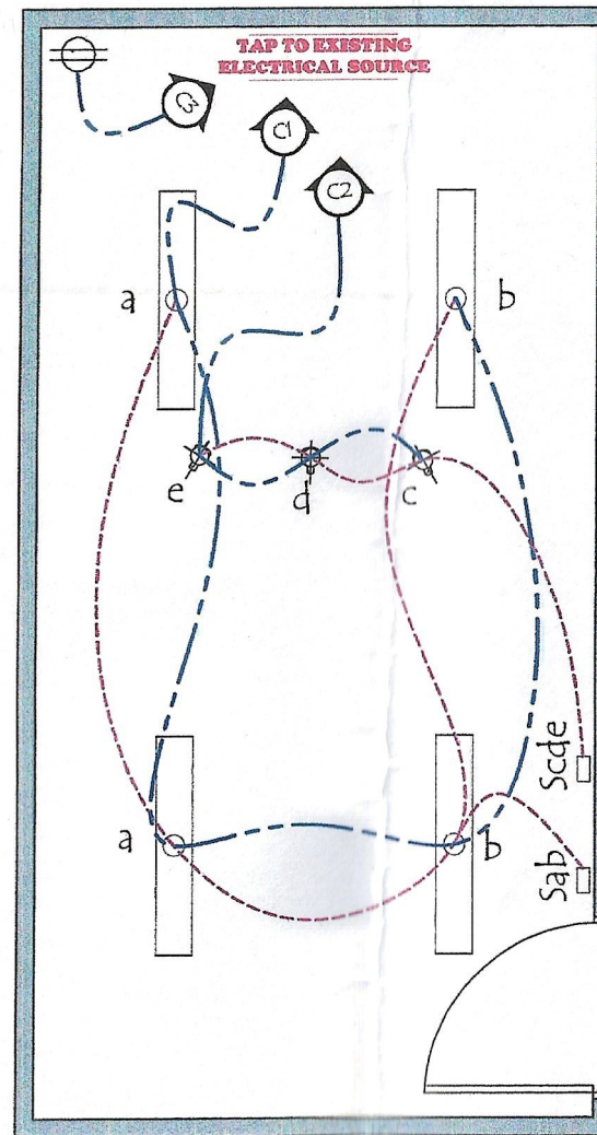
ELECTRICAL LAY-OUT SCALE: 24 : 1 M
