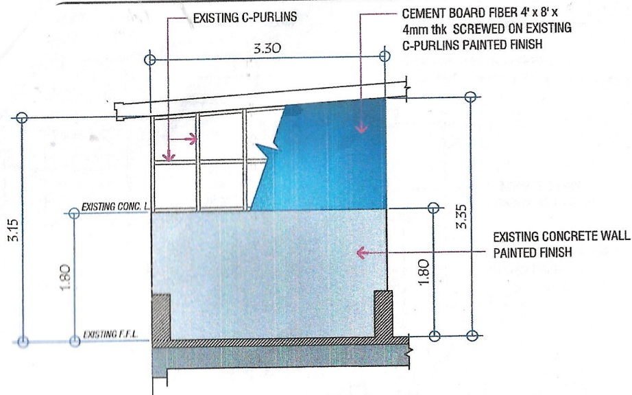
FRONT ELEVATION SCALE: 14 : 1 M
