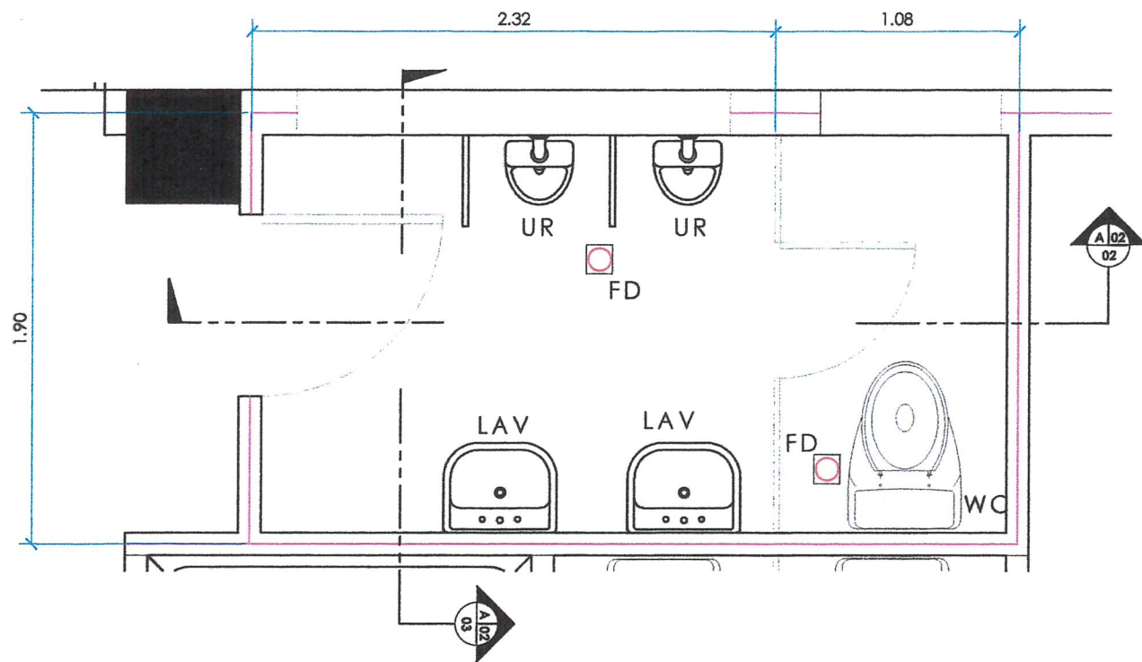
01 A-02 DETAIL PLAN (TOILET) SCALE : NTS
