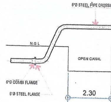
CANAL CROSSING SCALE: N.T.S.
