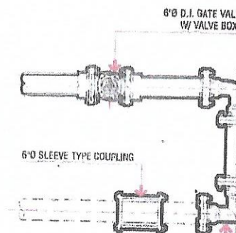
TAPPING POINT SCALE: N.T.S.
